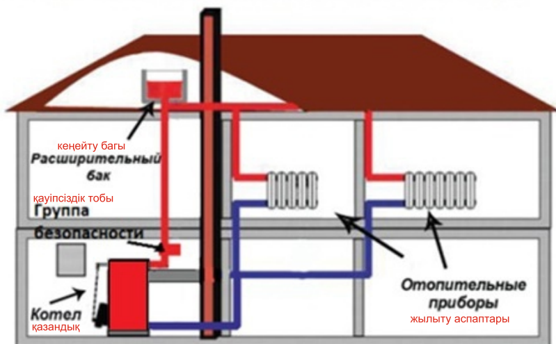
11 Сурет. Ашық кеңейту бағы бар жылыту жүйесін монтаждау / Рисунок 11. Монтаж системы отопления с открытым расширительным баком
