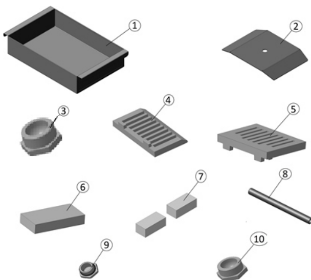
2 Сурет. Жеткізу жиынтығы / Рисунок 2. Комплект поставки
