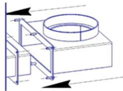
5-сурет. Ұластырғыны монтаждау / Рисунок 5. Монтаж переходника
