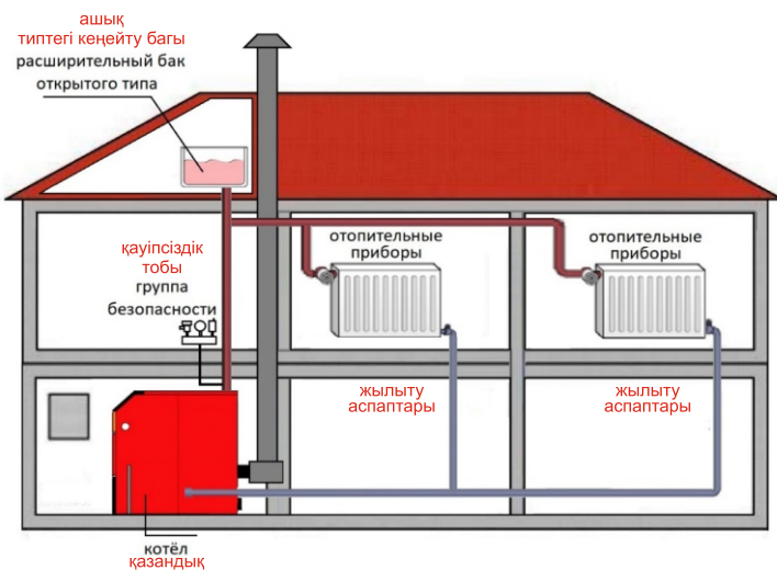
9 Сурет. Ашық кеңейту бағы бар жылыту жүйесін монтаждау / Рисунок 9. Монтаж системы отопления с открытым расширительным баком
