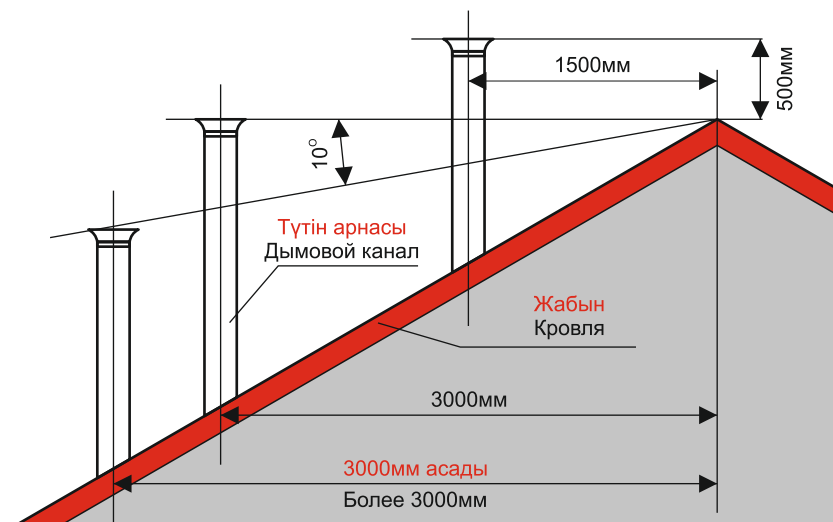
5-сурет. Мұржаны орнату тәсімі / Рисунок 5. Схема установки дымохода
