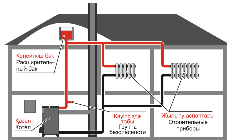
10-сурет. Кеңейткіш бағы ашық жылыту жүйесін монтаждау. / Рисунок 10. Монтаж системы отопления с открытым расширительным баком.
