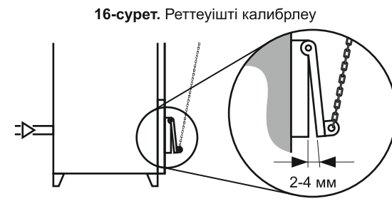
Рисунок 16. Калибровка регулятора
