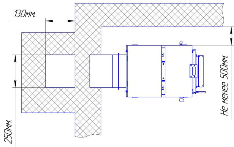
Рисунок 9. Схема установки котла (вид сверху)
