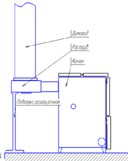
Рисунок 8. Схема соединения котла со стальной дымовой трубой
