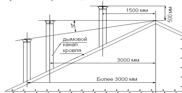
Рисунок 6. Схема установки дымохода
