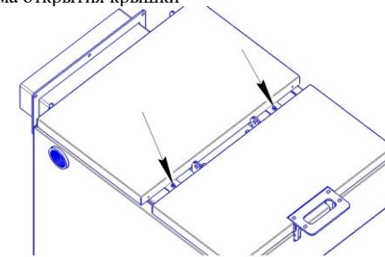
Рисунок 16. Схема открытия крышки
