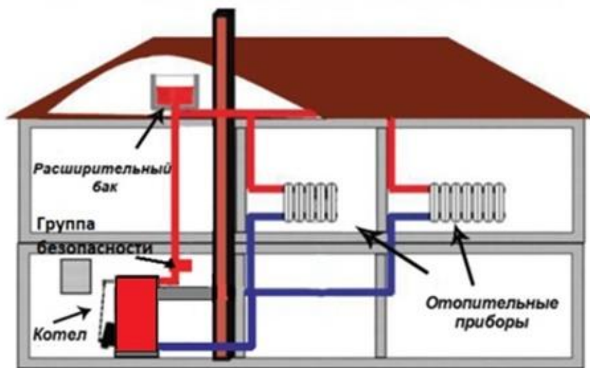
Рисунок 11. Монтаж системы отопления с открытым расширительным баком.
