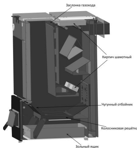
Рисунок 4. Внутреннее строение котла КС-Т 32
