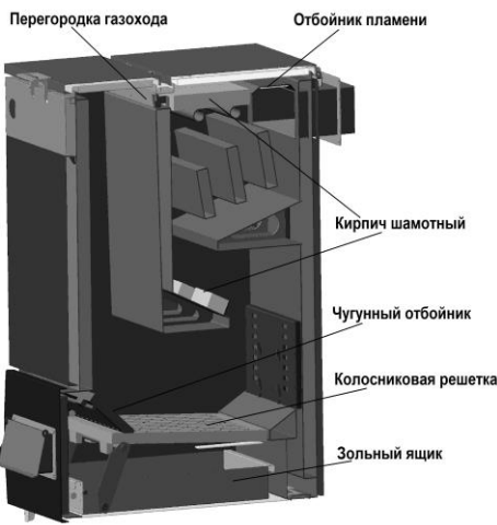
Рисунок 5. Внутреннее строение котла КС-Т 45
